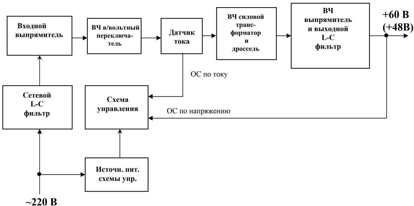
Рис.1. Структурная схема ИПС-950.
